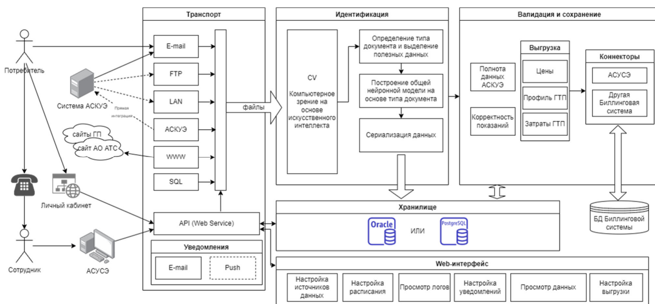
Рисунок 1 Структурная схема АИС Предбиллинг
