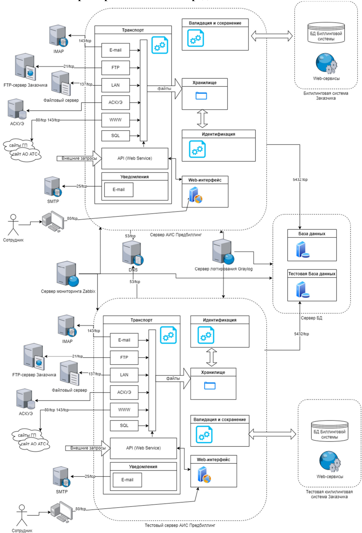
Рис.2 Схема развертывания АИС Предбиллинг в инфраструктуре предприятия
